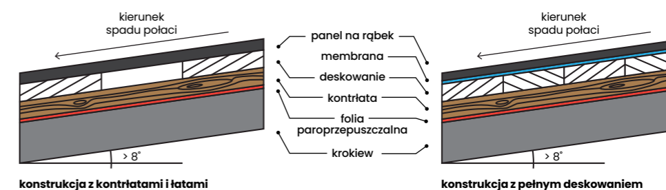
konstrukcja z kontrłatami i łatami
