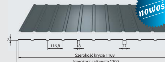
BLACHA TRAPEZOWA T14
